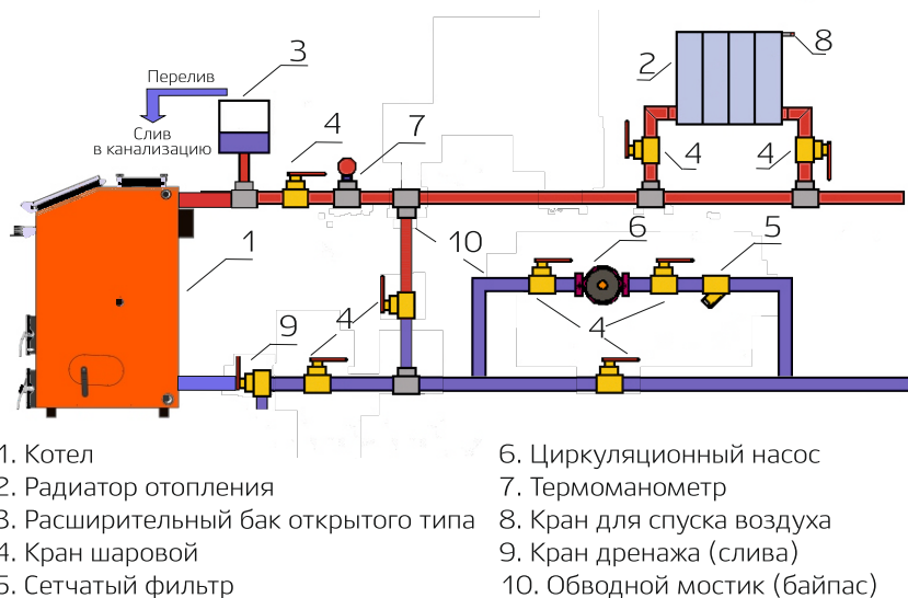
Рис. 9 Подключение котла к однотрубной открытой системе с принудительной циркуляцией теплоносителя
