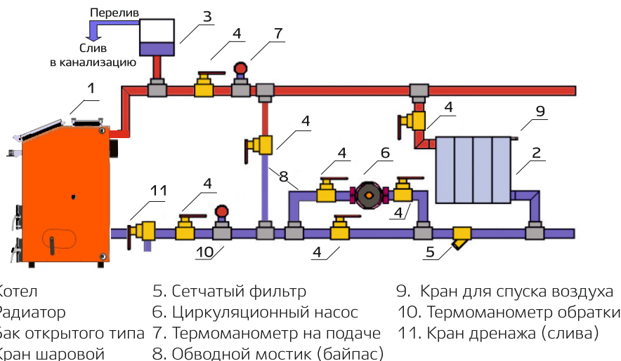
Рис. 8 Подключение котла к 2-х трубной открытой системе с принудительной циркуляцией теплоносителя
